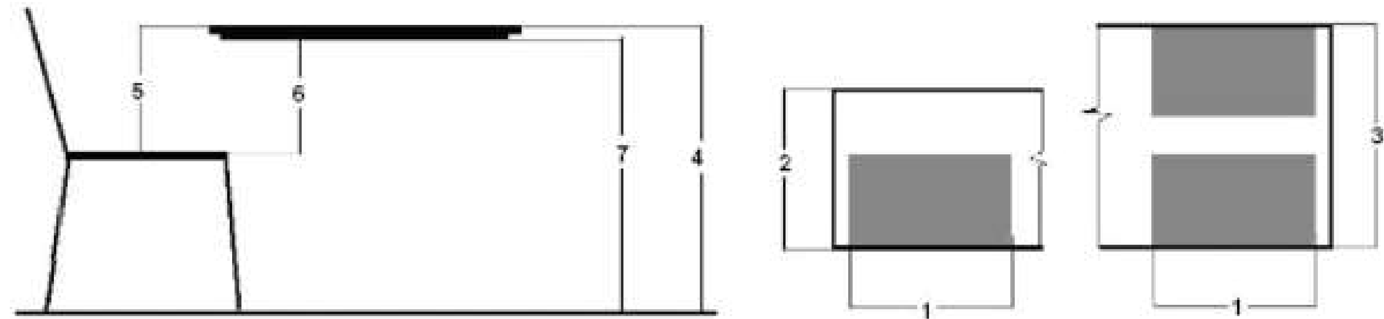
Obr. 1: Rozměry jídelních stolů dle normy ČSN 91 0820
