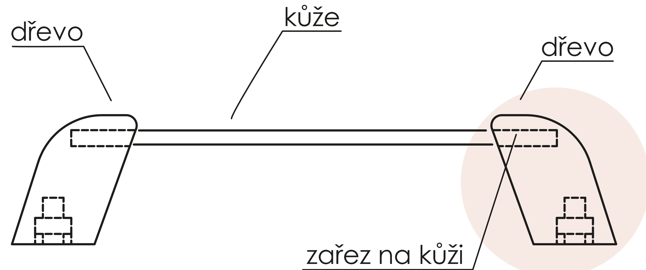
půdorys/ řez
