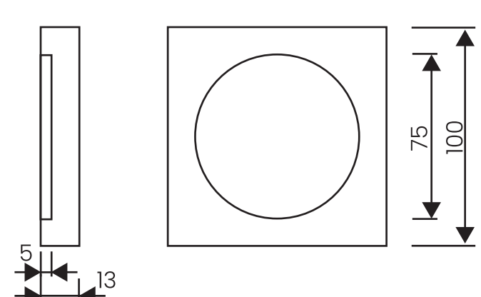
Rozměry produktu Jednotka: milimetry
