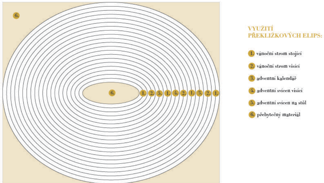
Obr. 187 Využití a rozvržení plochy materiálu
