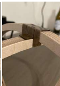
Obr. 158 Umístění mosazného kříže na překližkové obruče
