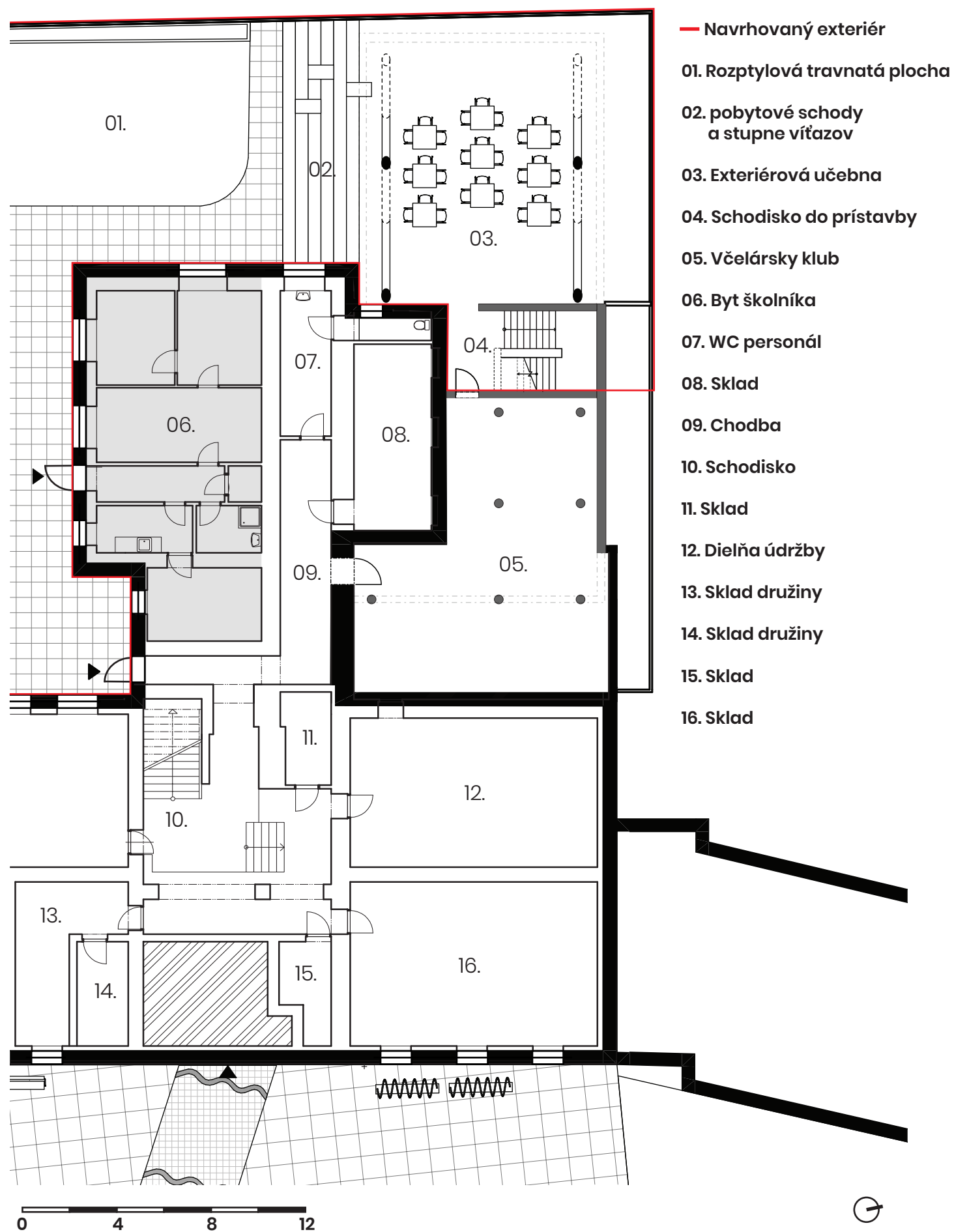
1. Základná škola Napajedla - Pôdorysné schéma 1. PP
