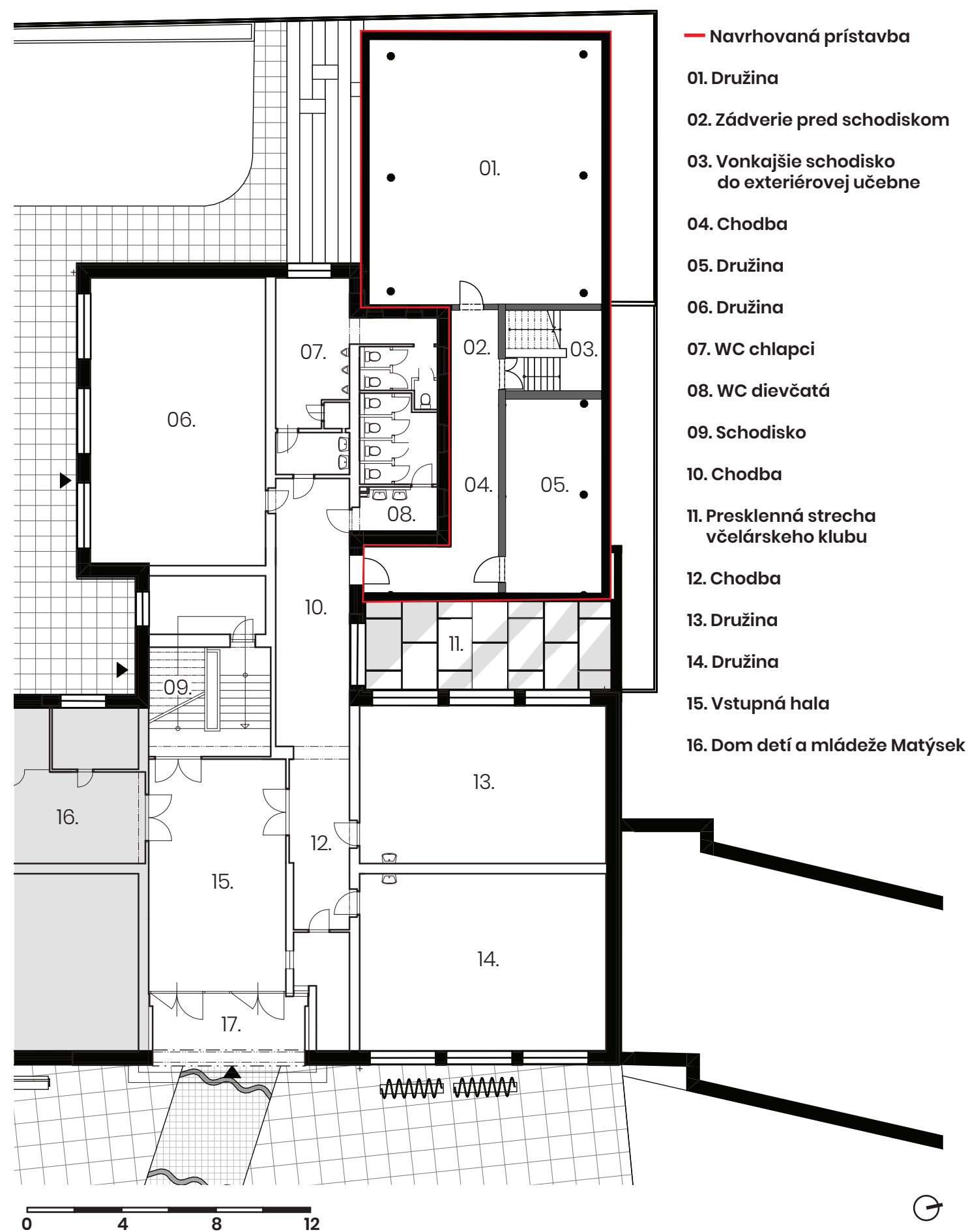
1. Základná škola Napajedla - Pôdorysné schéma 1. NP
