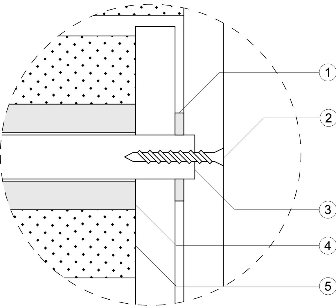
DETAIL A 1:1
