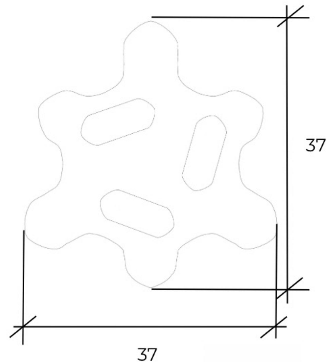
3. vrstva
